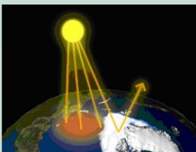
Albedo der Erde
