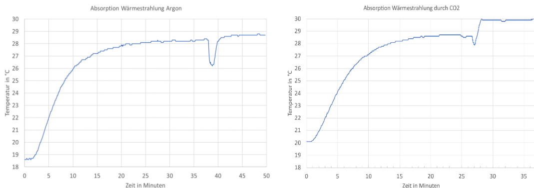
Abb. 5. Messwerte für die Temperatur innerhalb der Pappröhre, (links) vor und nach der Zugabe von Argon (links) und (rechts) vor und nach der Zugabe von \text{CO}_2 .
