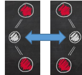
Abb. 6 Biegeschwingung eines \text{CO}_2 -Moleküls (Credits: Prof. Dr. B. Mayer)
