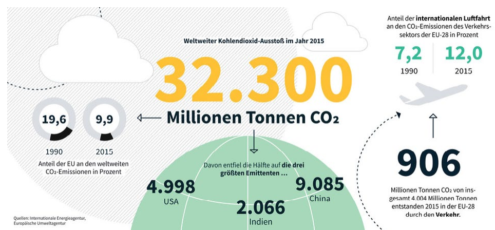
Abbildung 32 – Weltweiter Kohlendioxid-Ausstoß im Jahr 2015 (Credits: Internationale Energieagentur, Europäische Umweltsagentur)
