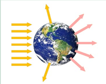
Die Erde wird von der Sonne bestrahlt und strahlt selbst
