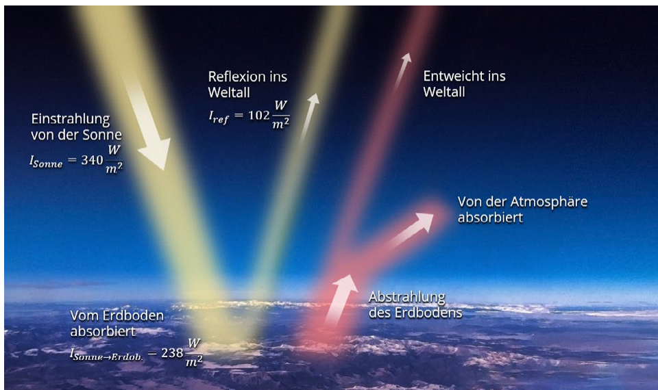
Abbildung 16 – Zwischenschritt zu einer Strahlungsbilanz mit Atmosphäre. (Credits: Strähle und Hohmann)
