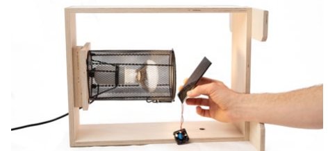
Einstrahlwinkel und Intensität
