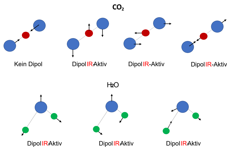
Abbildung 21 – IR-aktive Dipol-Moleküle (Credits: Scorza)
