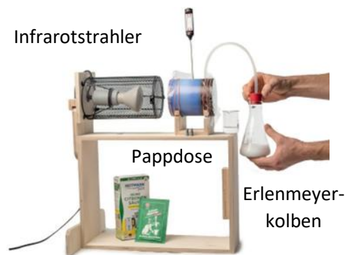
Experiment: Absorption von Wärmestrahlung
