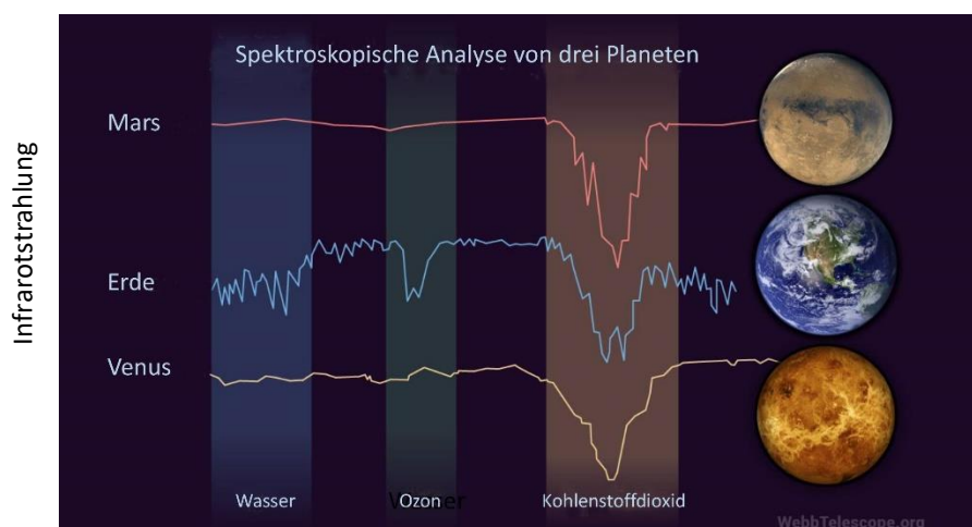
Abb. 7 Absorption von Infrarotstrahlung durch \text{CO}_2 durch planetare Atmosphären (Credits: WebTeleskop.org)
