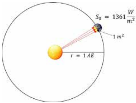
Abbildung 9 – Zur Messung der Solarkonstante bestimmt man die Leistung, die im Abstand Sonne-Erde auf 1m 2 Fläche auftrifft. (Credits: Scorza, Strähle)
