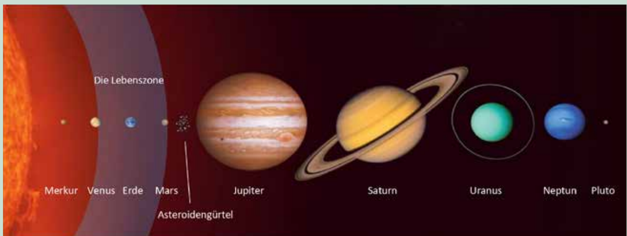
Die Planeten unseres Sonnensystems im Größenmaßstab. Die Abstände untereinander sind hier deutlich zu klein dargestellt! (Credits: Scorza)
