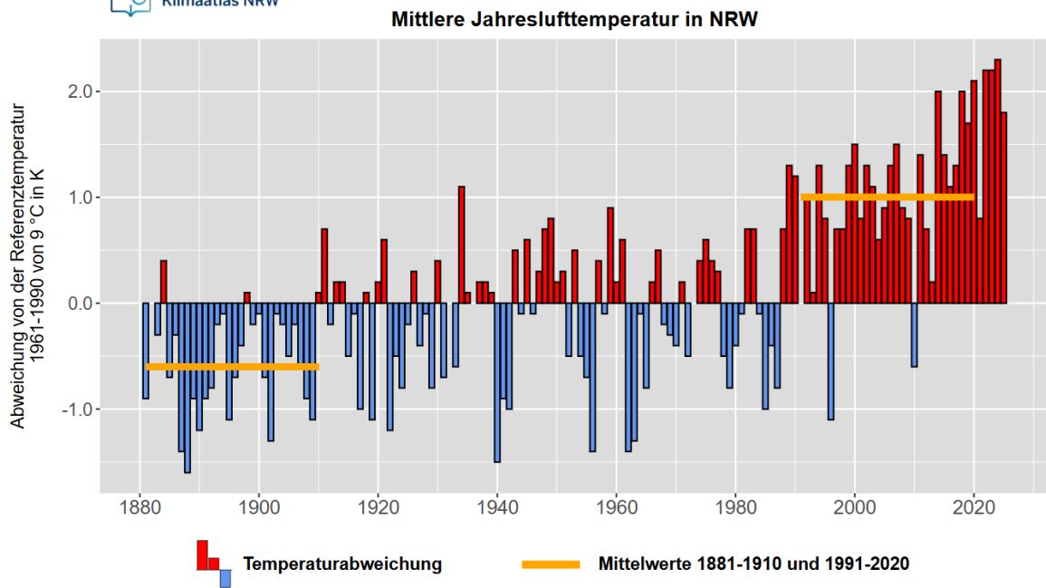
Abbildung 1b - Abweichungen von der Referenztemperatur (3)
