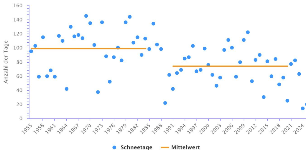
Abbildung 3 - Anzahl der Tage mit Schneedecke am Kahlen Asten (10)
