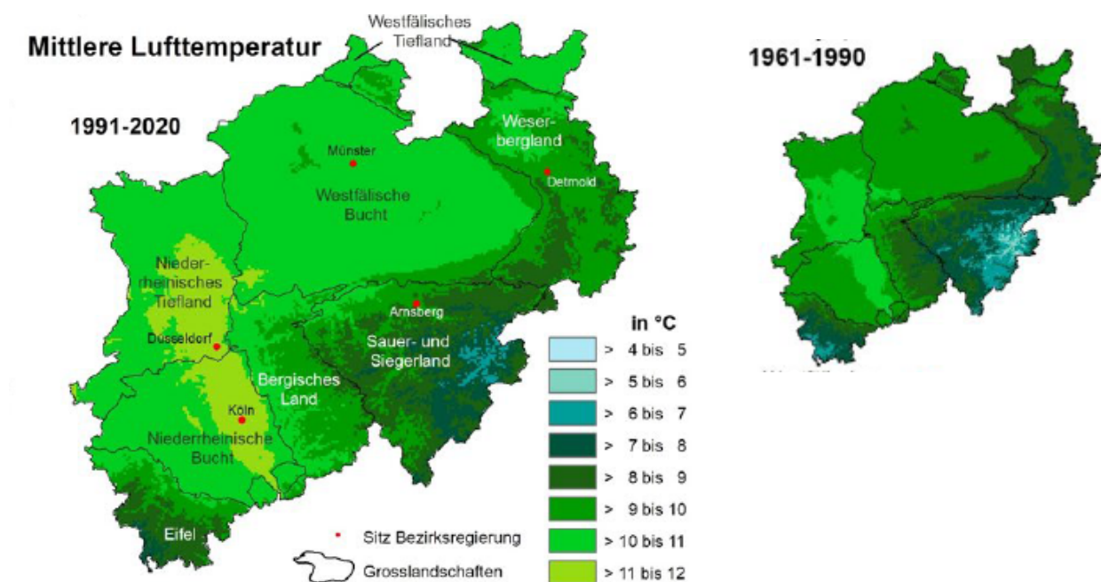
Abbildung 1a - Mittlere Lufttemperatur in NRW 1991-2020 im Vergleich zu 1961-1990 (3)
